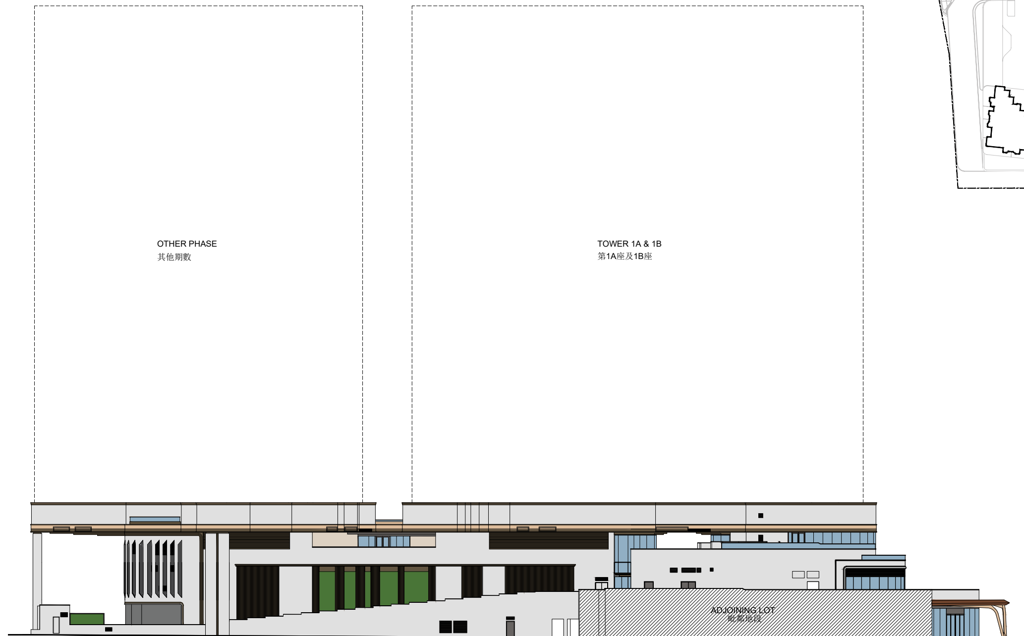
Podium Elevation Plan B 平台立面圖 B
