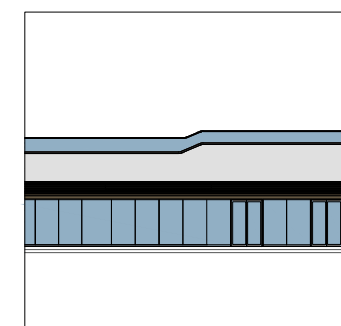
Podium Elevation Plan E 平台立面圖 E
